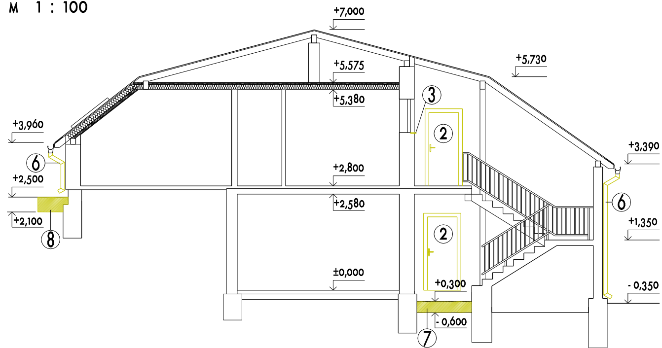
REZ A - A - BÚRACIE PRÁCE M 1 : 100
