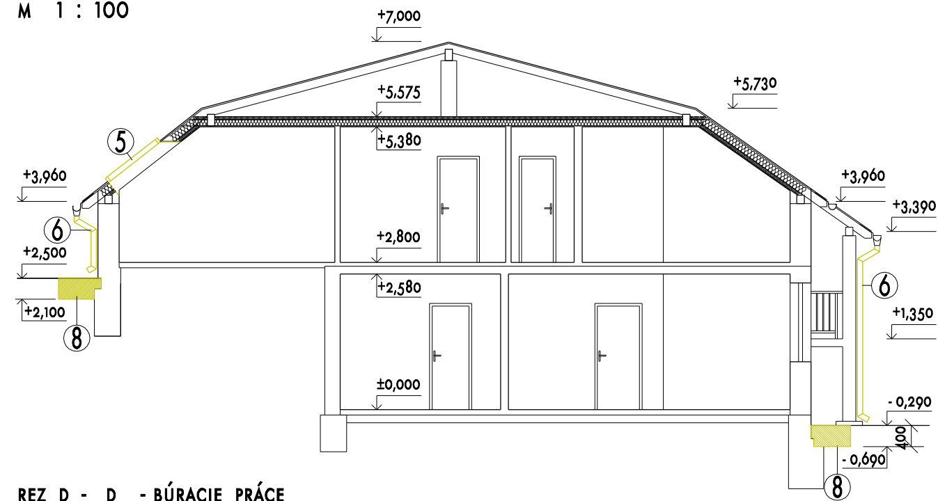
REZ B - B - BÚRACIE PRÁCE M 1 : 100
