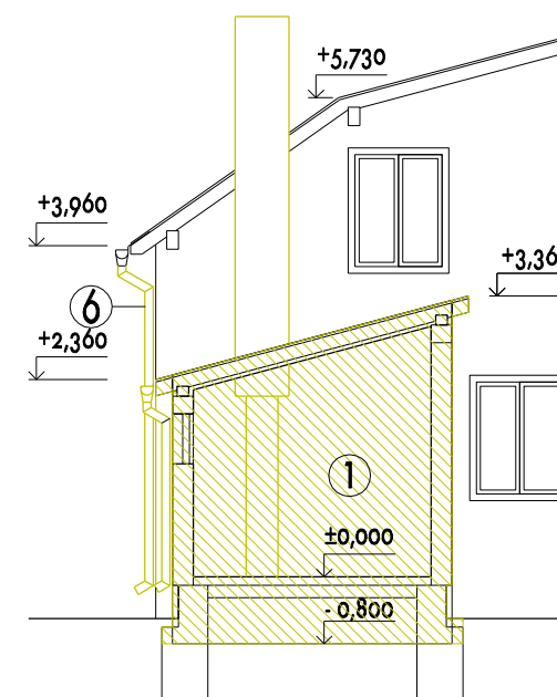
REZ D - D - BÚRACIE PRÁCE M 1 : 100
